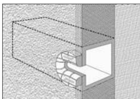
Schematický náčrt těžké budky, instalované ve vrstvě zateplení v atikovém prostoru objektu v místě stávajících VO
